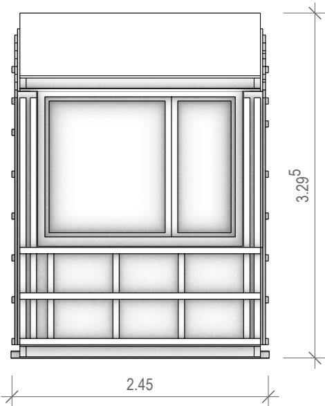
Ansicht EW-2
