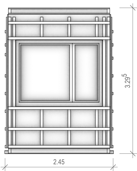
Ansicht EW-4
