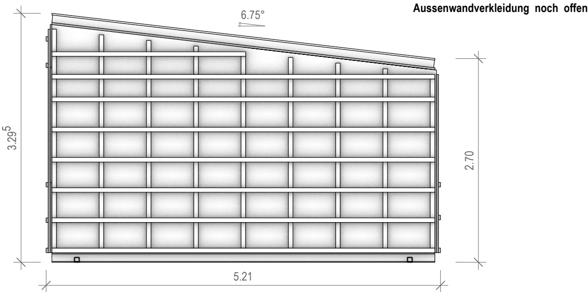
Ansicht EW-3
