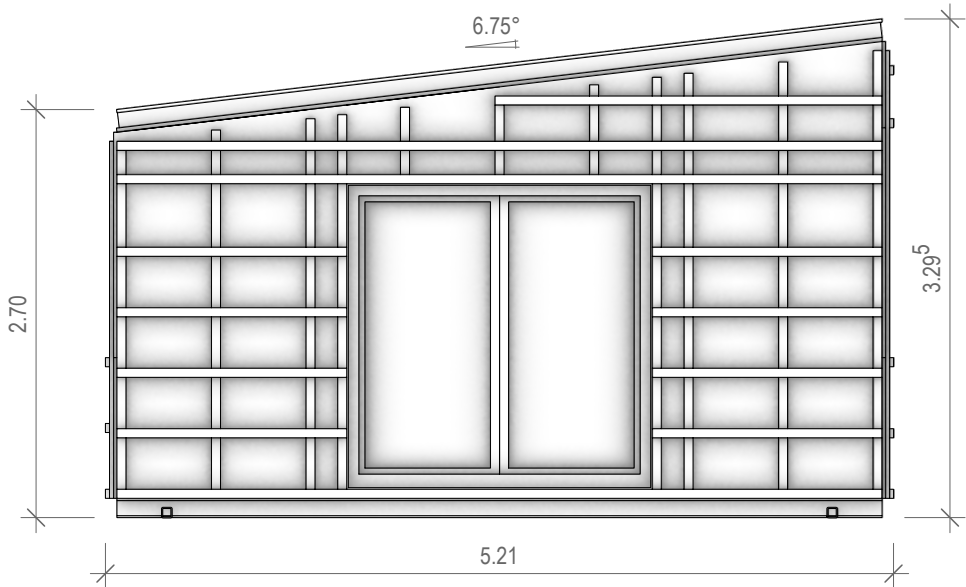
Ansicht EW-1
